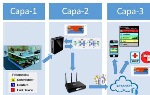
Fig. 2. Arquitectura del sistema de telemonitoreo y asistencia remota
